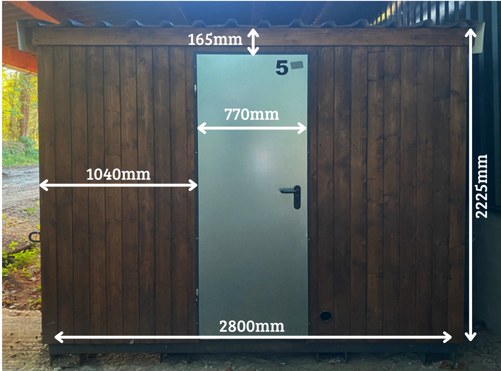
Rückansicht Verkaufsstand
