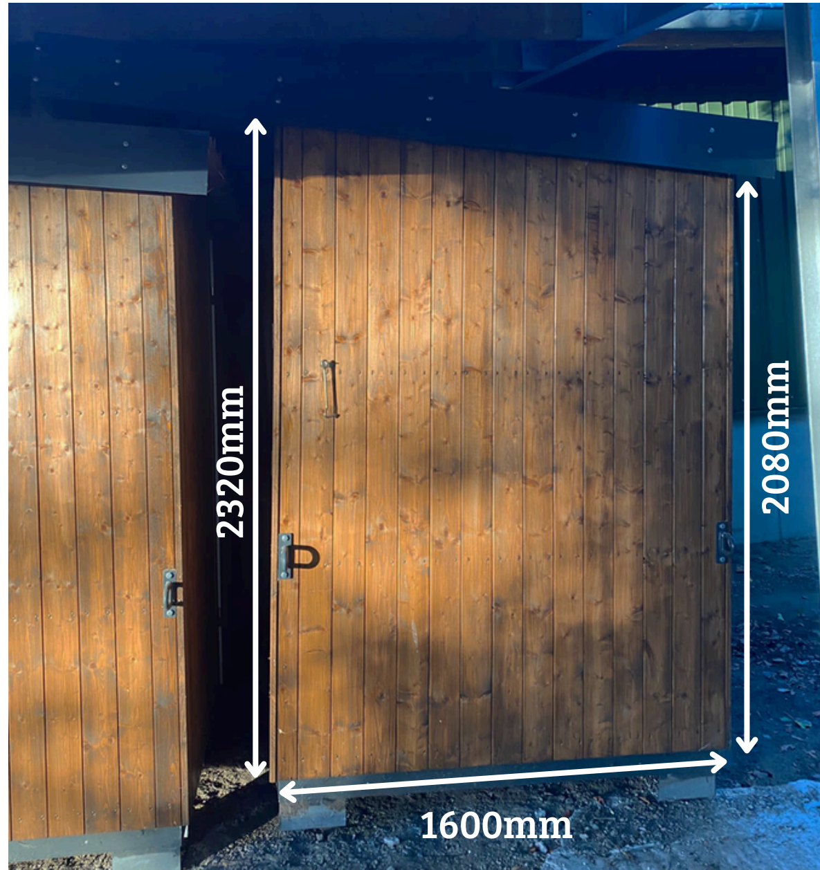
Seitenansicht Verkaufsstand
