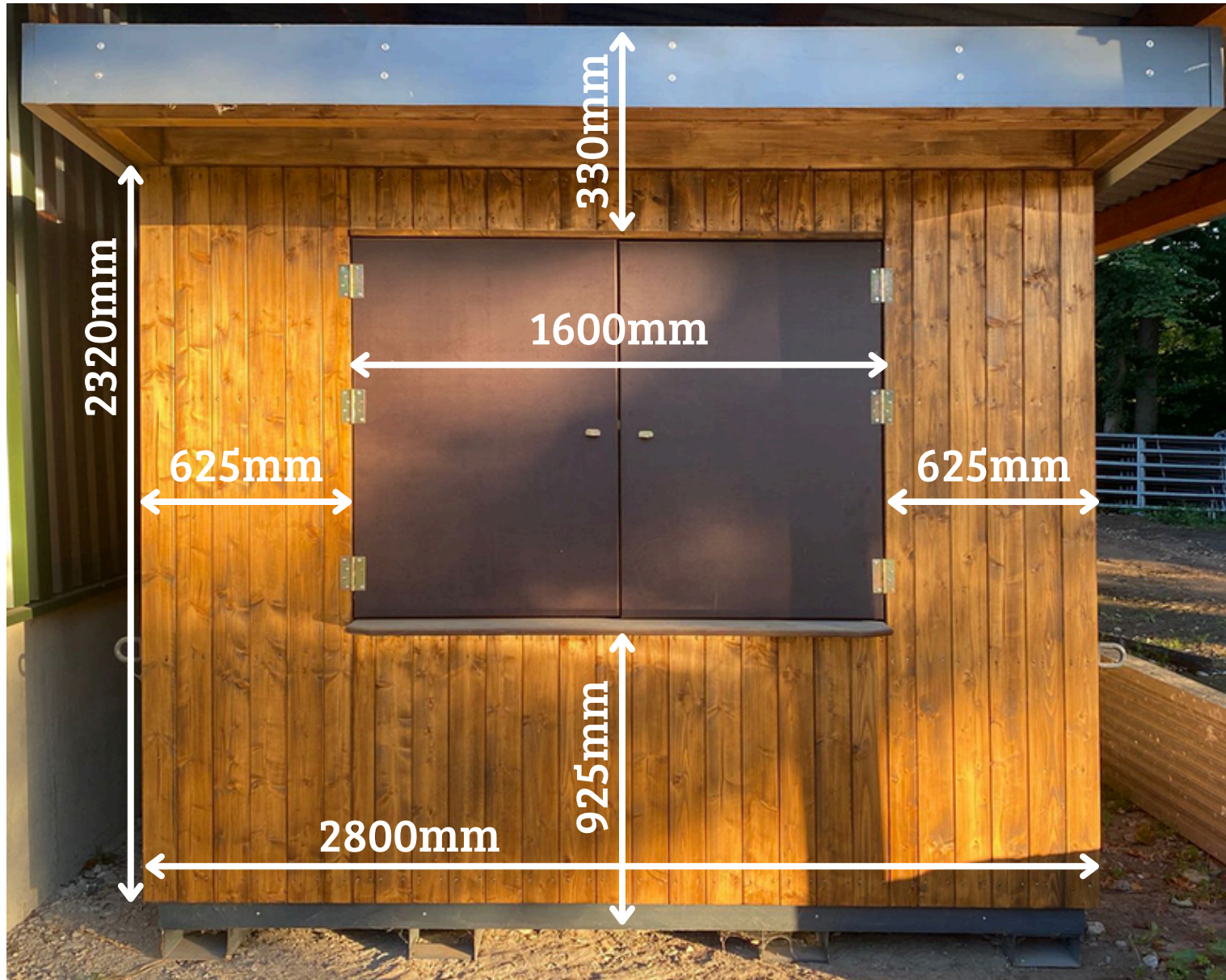
Frontansicht Verkaufsstand
